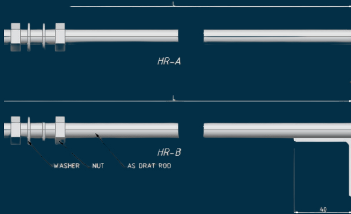
HANGER ROD
