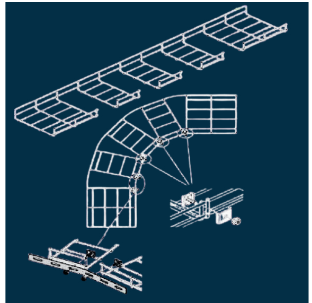
ELBOW LONG 90'
